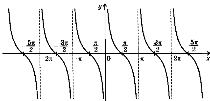
график — котангенсоида
