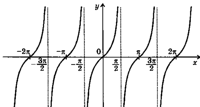
график — тангенсоида
