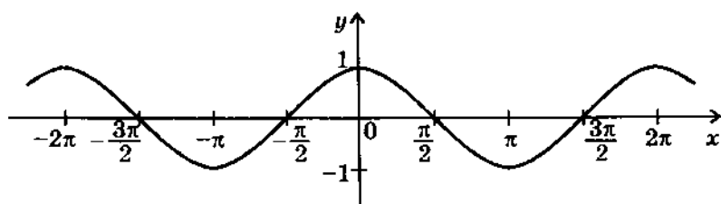
график — косинусоида
